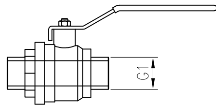
Kugelhahn/Außengewinde
